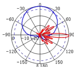
1710-2490MHz: \pm 45^\circ Pol.
