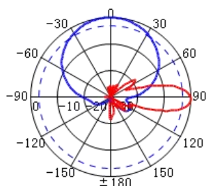
690-960MHz: \pm 45^\circ Pol.
